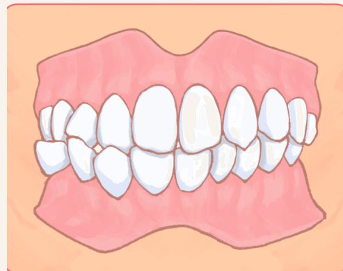
交叉咬合
